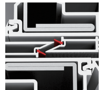
4중 기밀구조 여밈대 부분 4중 기밀구조 적용으로 기밀성 강화
