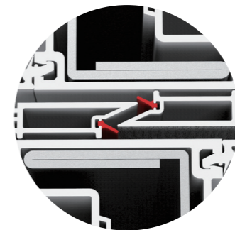
4 4중 기밀구조 어림대 부분 4중 기밀구조 적용으로 기밀성 강화
